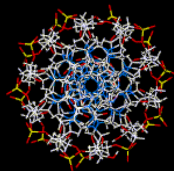
B-DNA
