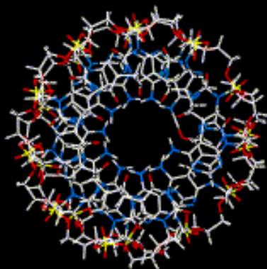
A-DNA
